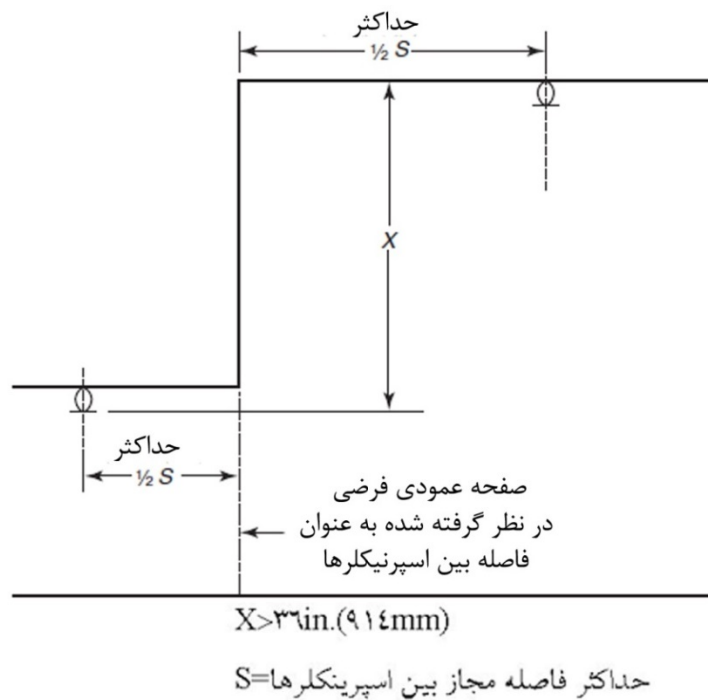
شکل ۸-۶-۴-۱-۳-الف - تغییر عمودی در ارتفاع سقف بزرگتر از 914 \text{ mm (36 in.)}
