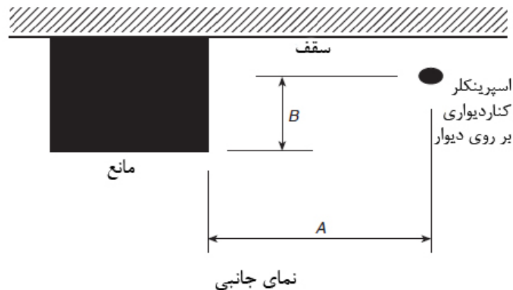
شکل ۸-۷-۵-۱-۴- جانمایی اسپرینکلرها برای جلوگیری موانع در امتداد دیوار (اسپرینکلرهای اسپری کننده دیواری مسکونی)
