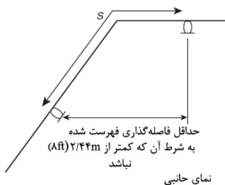
شکل ۸-۱۰-۳-۶-ب- حداقل فاصله بین اسپرینکلرها با سقف‌های شیب‌دار- چیدمان ب
