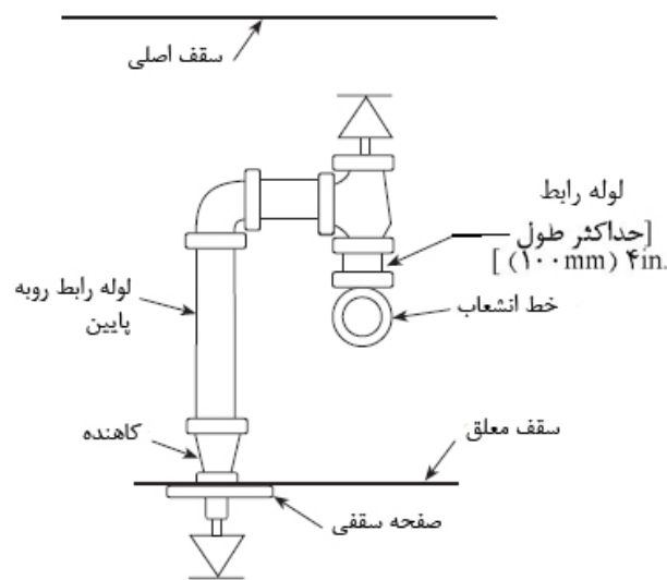
شکل ۳-۴-۲۰-۱۵-۸- اسپرینکلرها در فضاهای پنهان و زیر سقف
