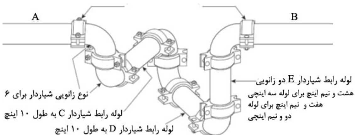
شکل ۹-۳-۳-۴- مجموعه جداساز لرزه‌ای با فاصله جداسازی ۲۰۰mm (۸in.) در محل تقاطع لوله‌ها با قطر اسمی تا ۱۰۰mm (۴in.). (برای سایر فواصل جداسازی و اندازه لوله‌ها، طول‌ها و فواصل باید متناسباً اصلاح شوند)
