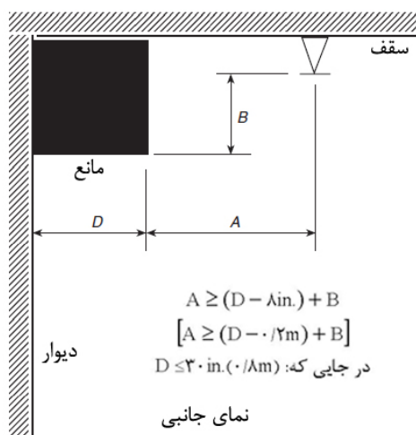
شکل ۸-۸-۵-۱-۲-ب- موانع در مقابل دیوارها (اسپرینکلرهای اسپری‌کننده بالازن و پایین‌زن پوشش گسترده)
