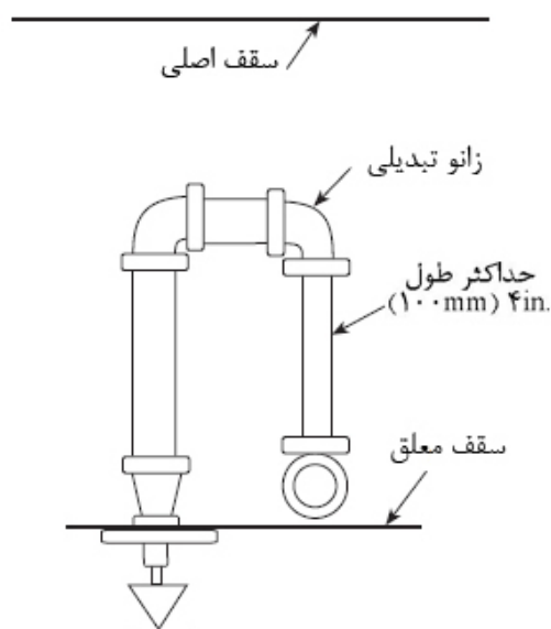
شکل ۲-۴-۲۰-۱۵-۸- لوله رابط و زانویی کاهنده تغذیه اسپرینکلر زیر سقف
