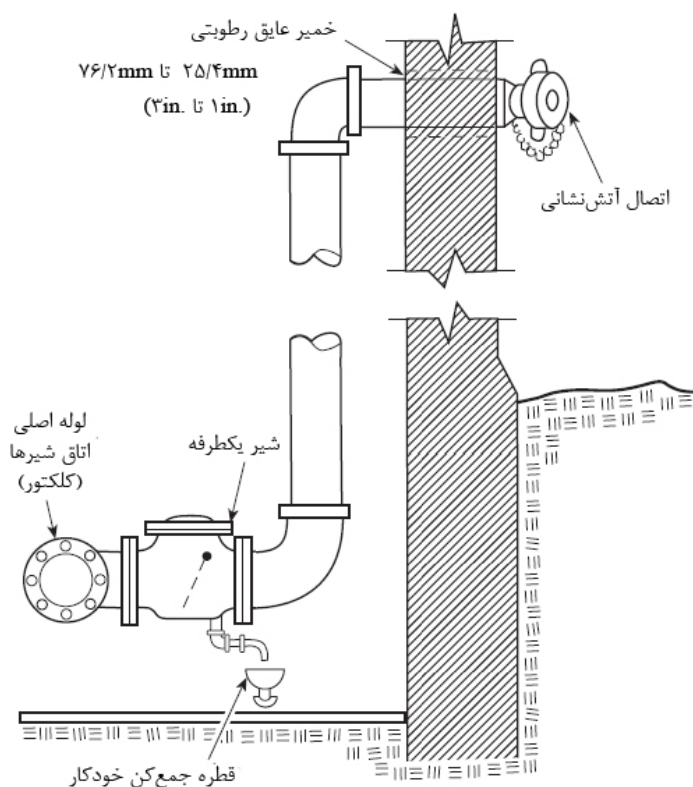
شکل ۸-۱۷-۲-۱- اتصال آتش‌نشانی
