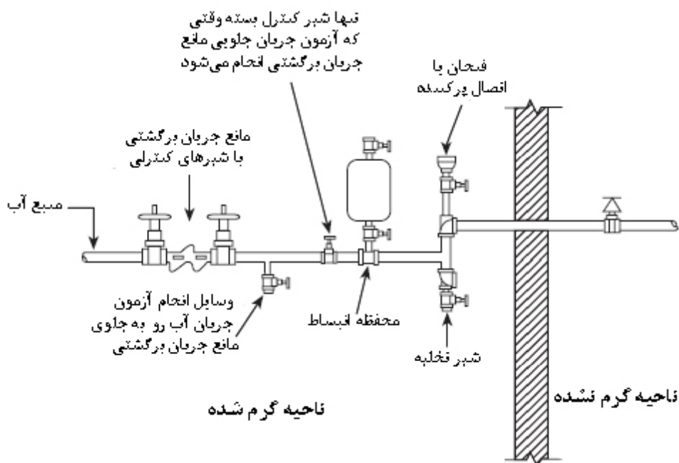
شکل ۷-۶-۳-۳- آرایش لوله‌کشی به همراه ابزار جریان برگشتی
