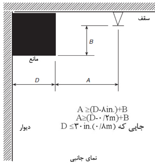
شکل ۸-۱۰-۶-۱-۲-ب- موانع مقابل دیوار (اسپرینکلرهای اسپری کننده بالازن و پایین زن مسکونی)
