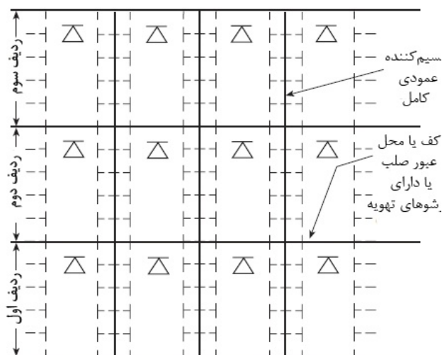
شکل ۸-۵-۱۰ الف- اسپرینکلرها در قفسه‌های کتاب چندردیفی با تقسیم‌کننده‌های عمودی کامل
