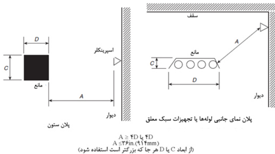
شکل ۸-۹-۵-۱-۴- حدافل فاصله از موانع (اسپرینکلرهای اسپری کننده دیواری پوشش گسترده)
