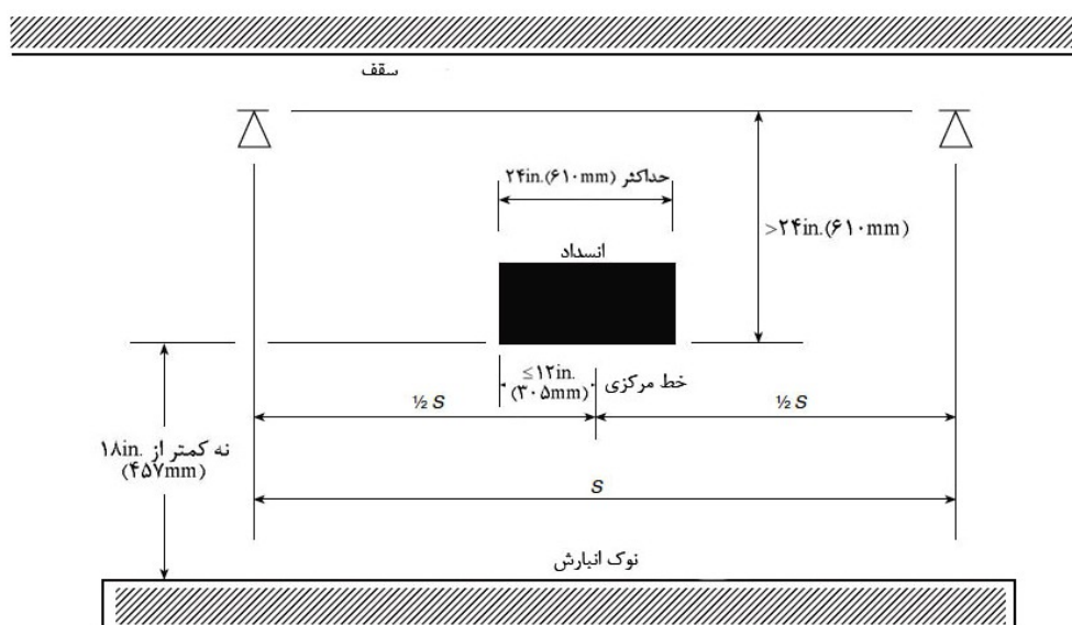
شکل ۸-۱۱-۵-۳ مانع بزرگتر از 24\text{in.} ( 610\text{mm} ) زیر اسپرینگلر (اسپرینگهای CMSA)
