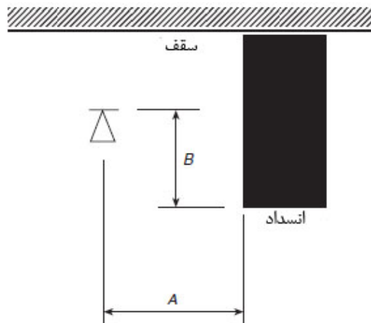
شکل ۸-۱۱-۵-۲-۱-۲ جانمایی اسپرینکلر از مانع برای جلوگیری از تاثیر آن بر تخلیه آب (اسپرینکلرهای CMSA)
