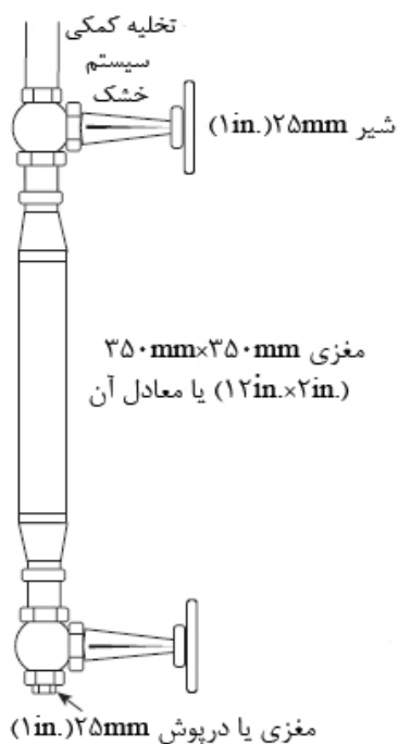
شکل ۵-۳-۵-۲-۱۶-۸- تخلیه کمکی سیستم خشک
