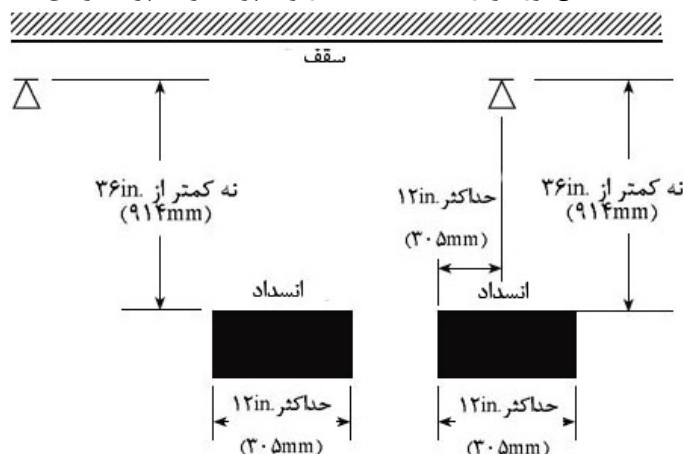
شکل ۸-۱۱-۵-۳ مانع بزرگتر از 36\text{in.} ( 914\text{mm} ) زیر اسپرینگلر (اسپرینگهای CMSA)
