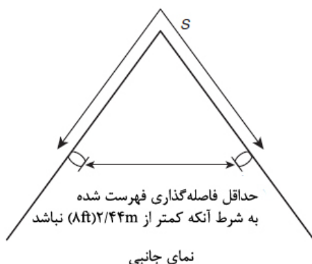
شکل ۸-۱۰-۳-۶-الف- حداکثر فاصله بین اسپرینکلرها با سقف‌های شیب‌دار- چیدمان الف
