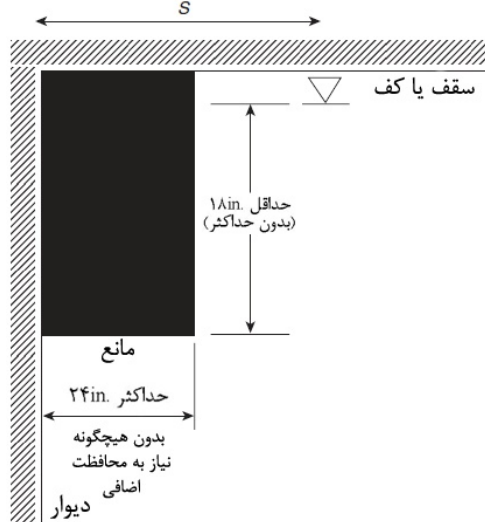
شکل ۸-۸-۵-۱-۲-پ- موانع در مقابل دیوارها (اسپرینکلرهای اسپری‌کننده بالازن و پایین‌زن پوشش گسترده)
